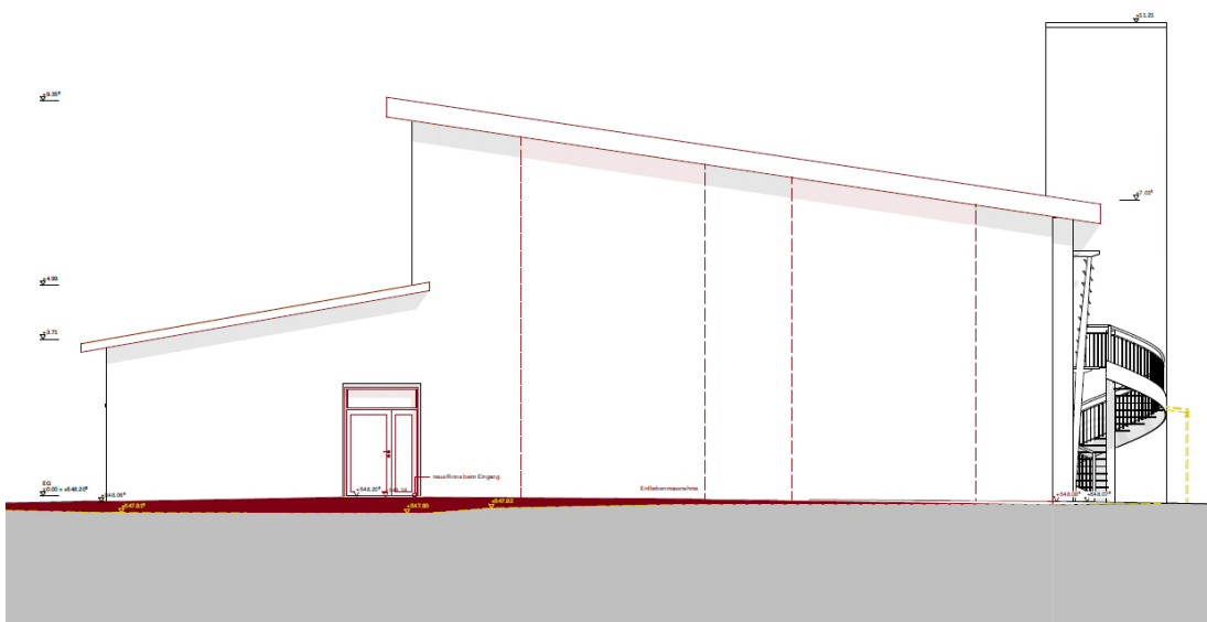
Nordwestfassade
