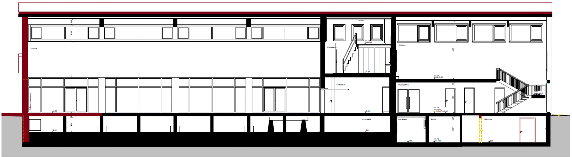
Längsschnitt
