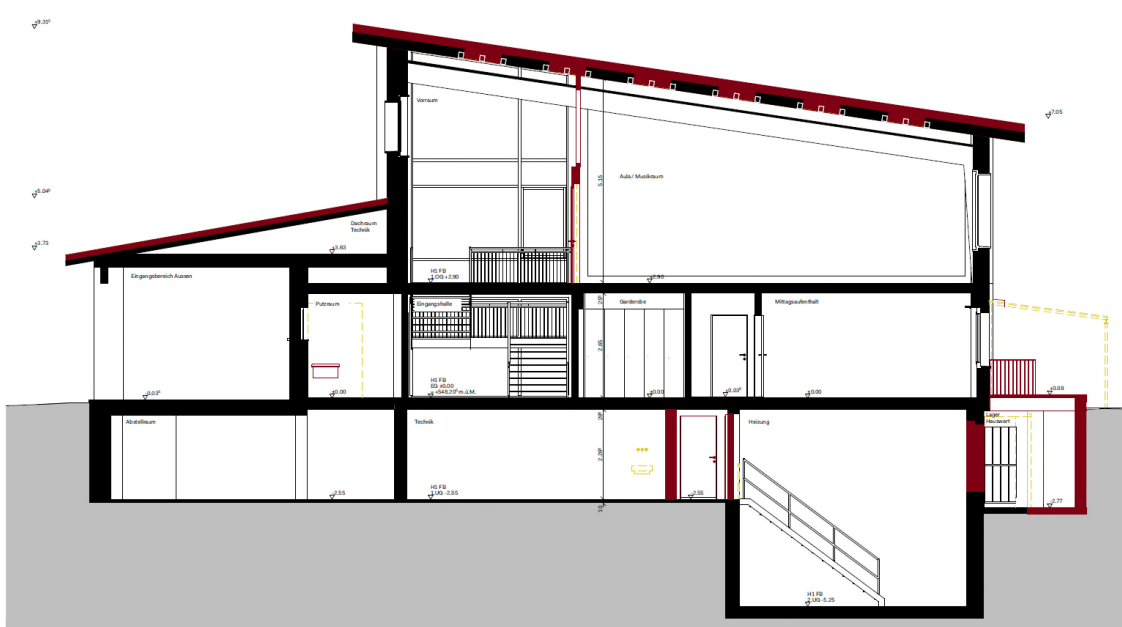
Querschnitt Aula
