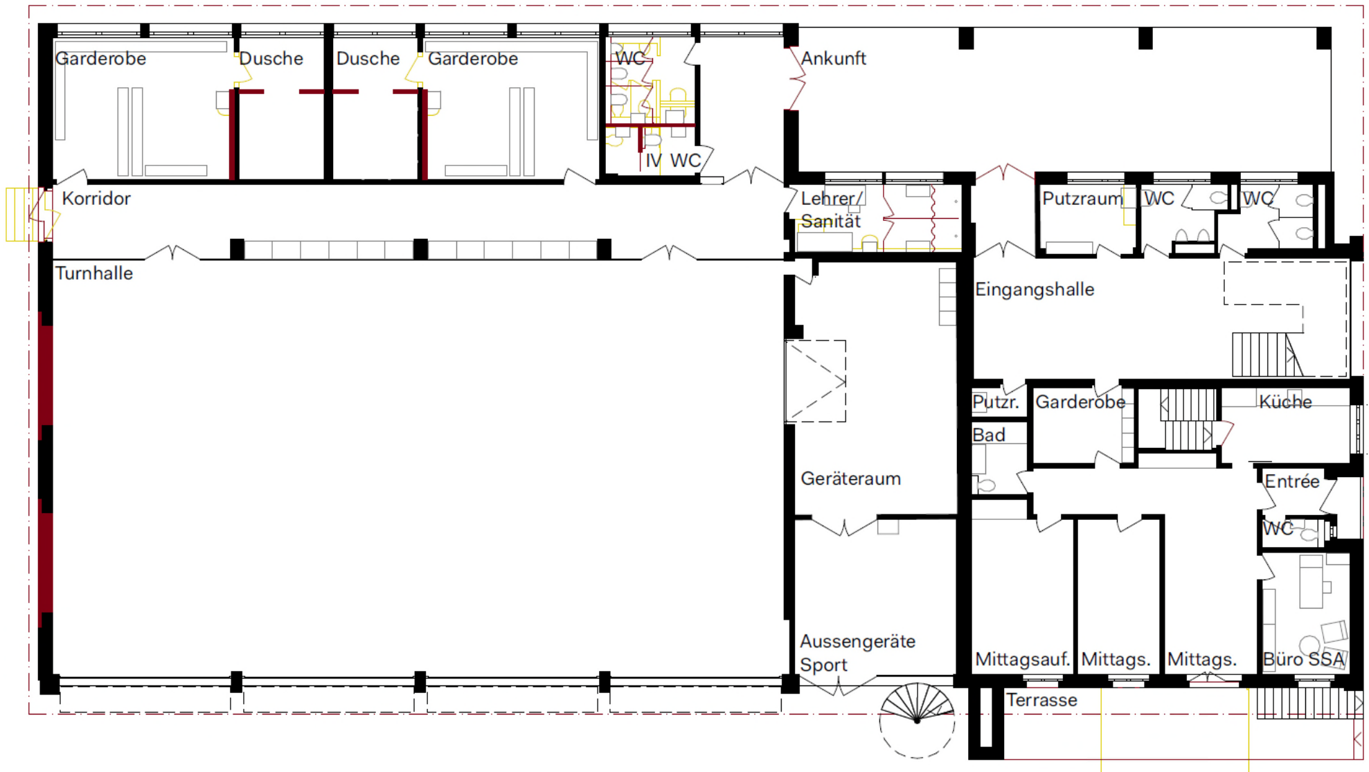
Grundriss Erdgeschoss
