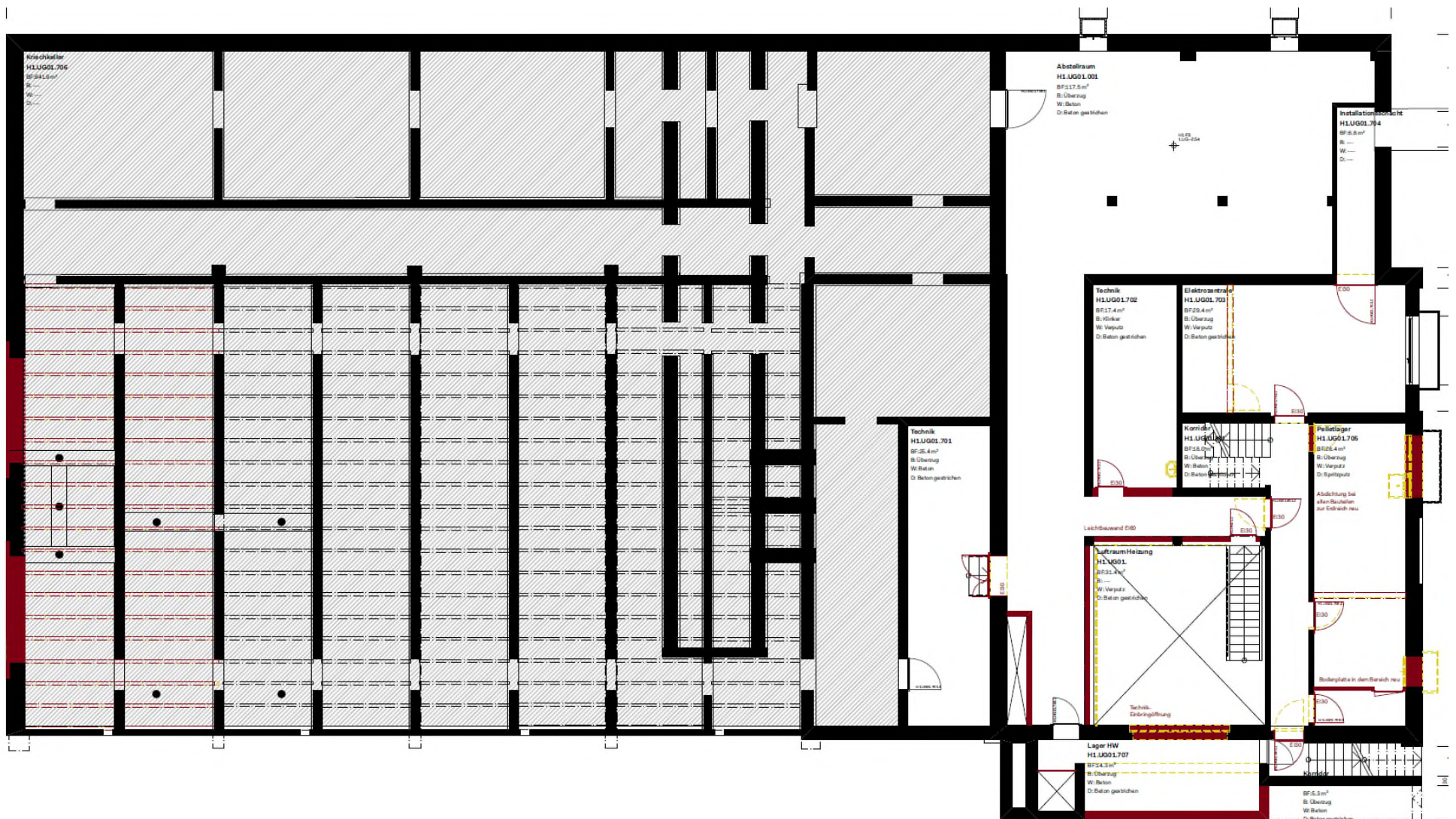
Grundriss Untergeschoss
