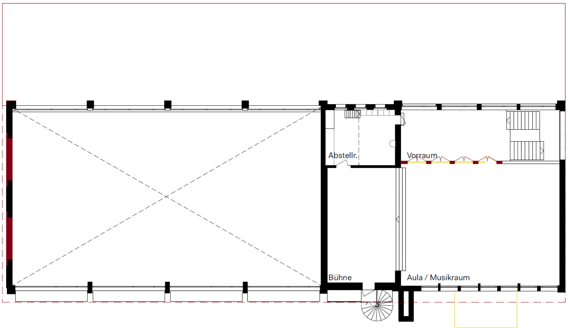
Grundriss Obergeschoss
