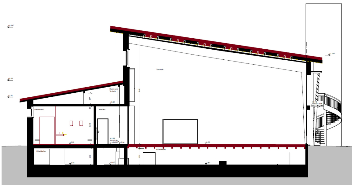
Querschnitt Turnhalle
