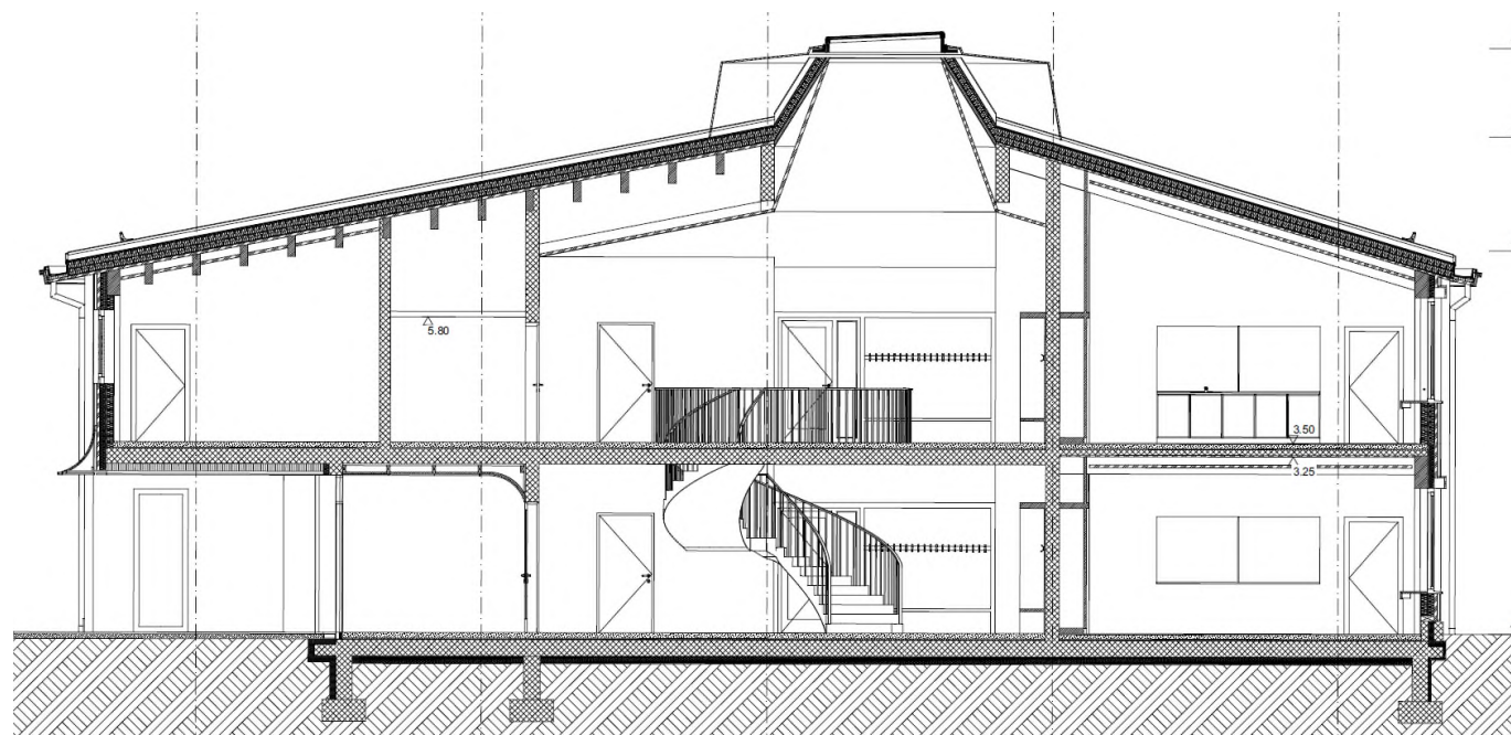
Querschnitt C-C
