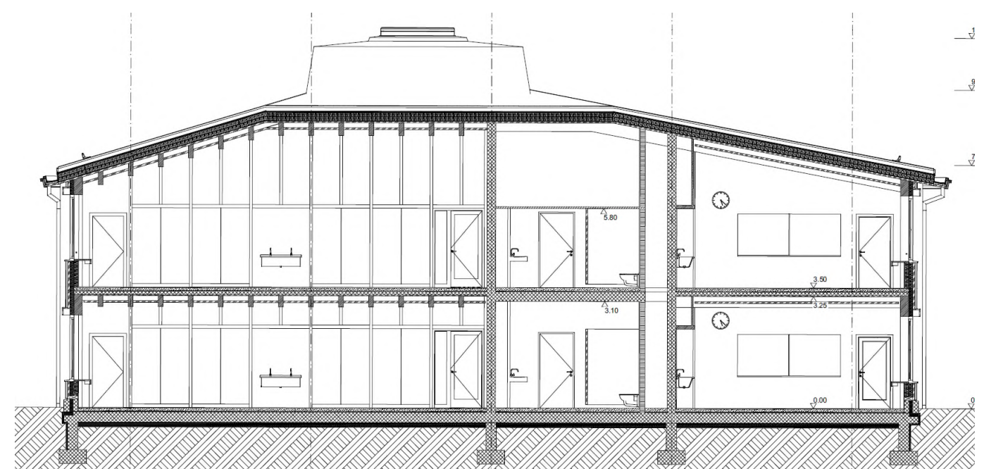
Querschnitt D-D
