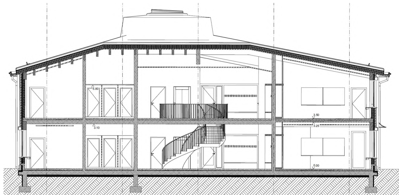
Querschnitt A-A
