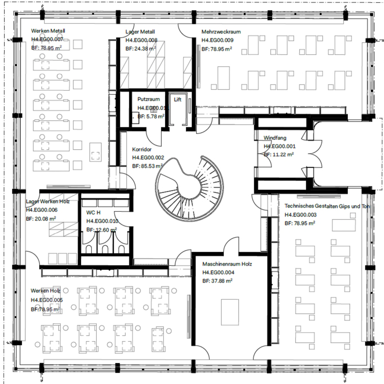
Grundriss Erdgeschoss
