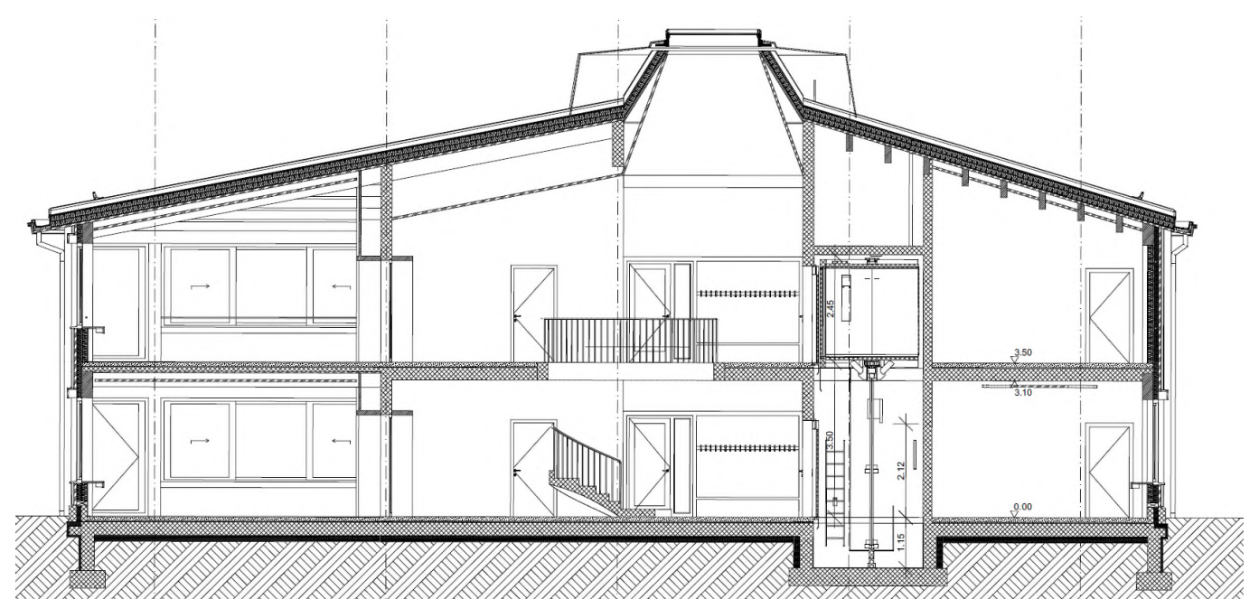
Querschnitt B-B
